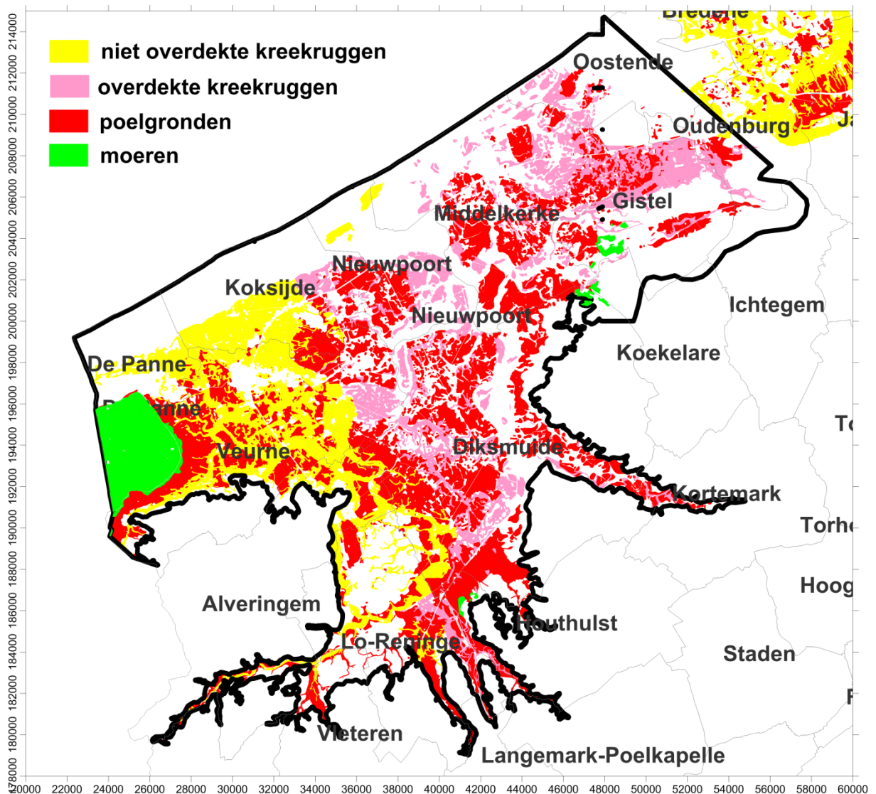
Figuur 2.10 Ligging van de kreekgruggen en poelgronden in het studiegebied op basis van de bodemkaart (samenstelling van bovenste 1.25 m).
