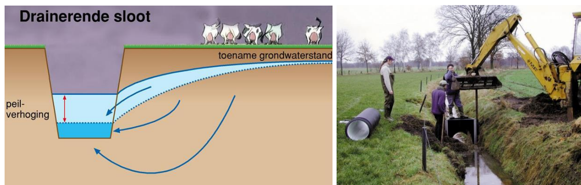
Figuur 3.7 Waterconservering door stuwtjes door het langer vasthouden van grondwater (De Louw et al., 2001).
