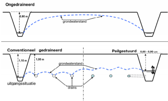
Fig. 1.1 Dwarsdoorsneden van een perceel: ongedraineerd (boven), conventioneel (CD; onder links) en peilgestuurd (PD) gedraineerd (onder rechts).
