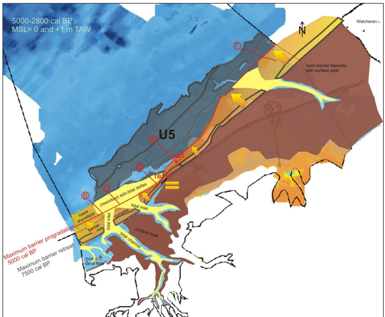
Figuur 2.4. Paleogeografische reconstructie van de kustvlakte, ongeveer 5000 à 2800 jaar geleden (Mathys (2009) in combinatie met Baeteman (2005)). De zeespiegel evolueerde in die tijdspanne van 0 tot +1 m TAW. In het westelijk kustgebied zijn er twee grote zeegaten, één bij de monding van de paleovallei van de IJzer en één ter hoogte van de huidige monding van de IJzer. Het paleo-zeegat in het oostelijk kustgebied is gelegen voor het huidige Zeebrugge.
